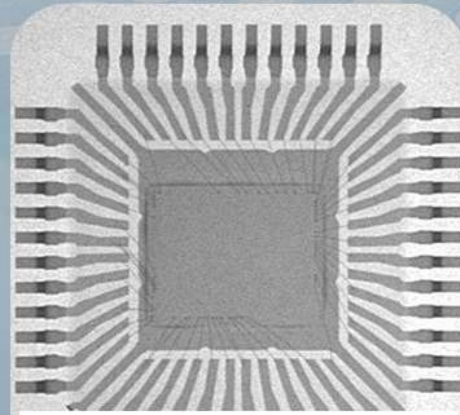
X-ray 검사
