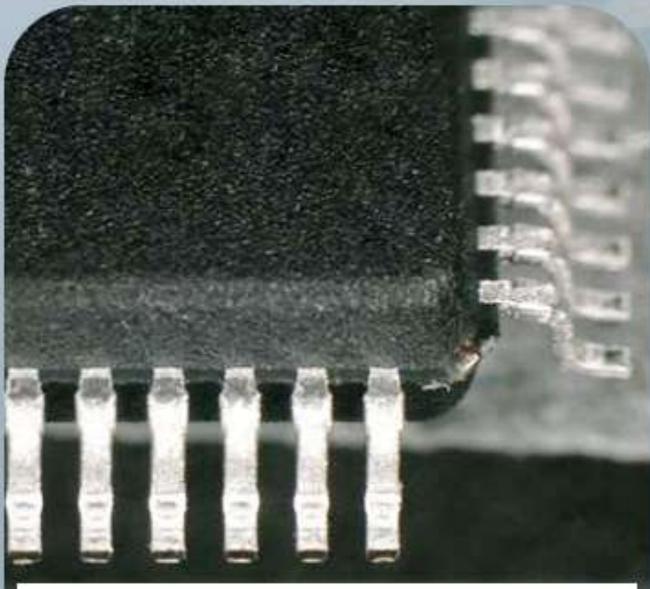
반도체 외관검사
